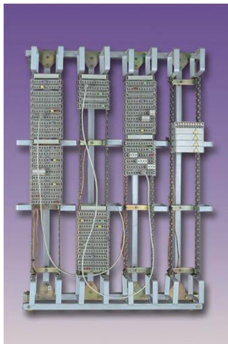
Рис.2 Каркас настенный односторонний на рейках.
